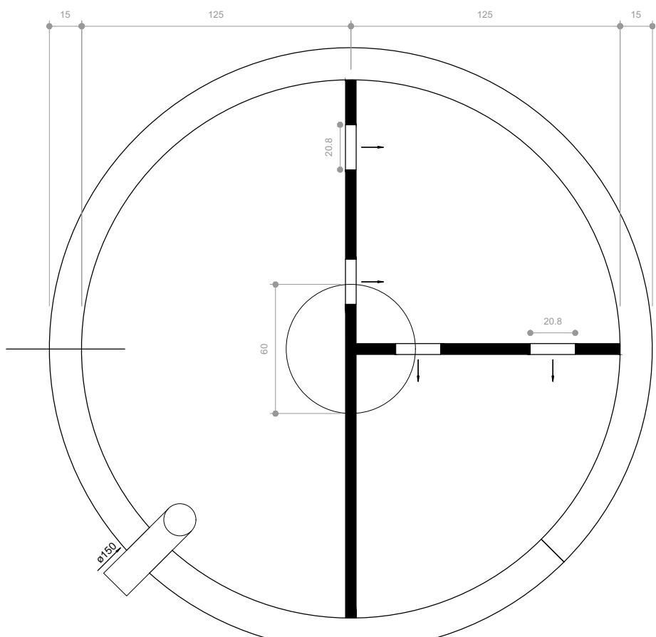
TANQUE SÉPTICO PLANTA BAIXA - ESC. 1:25
