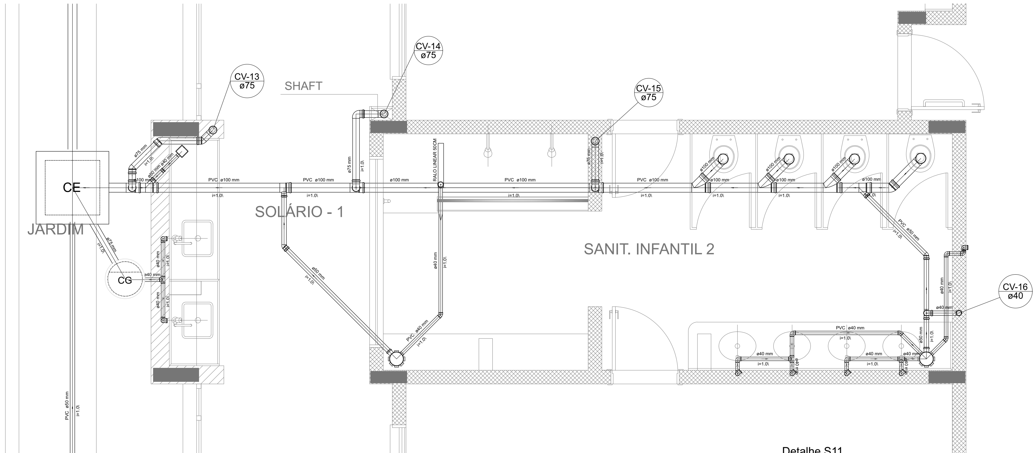
Detalhe S11 escala 1:25
