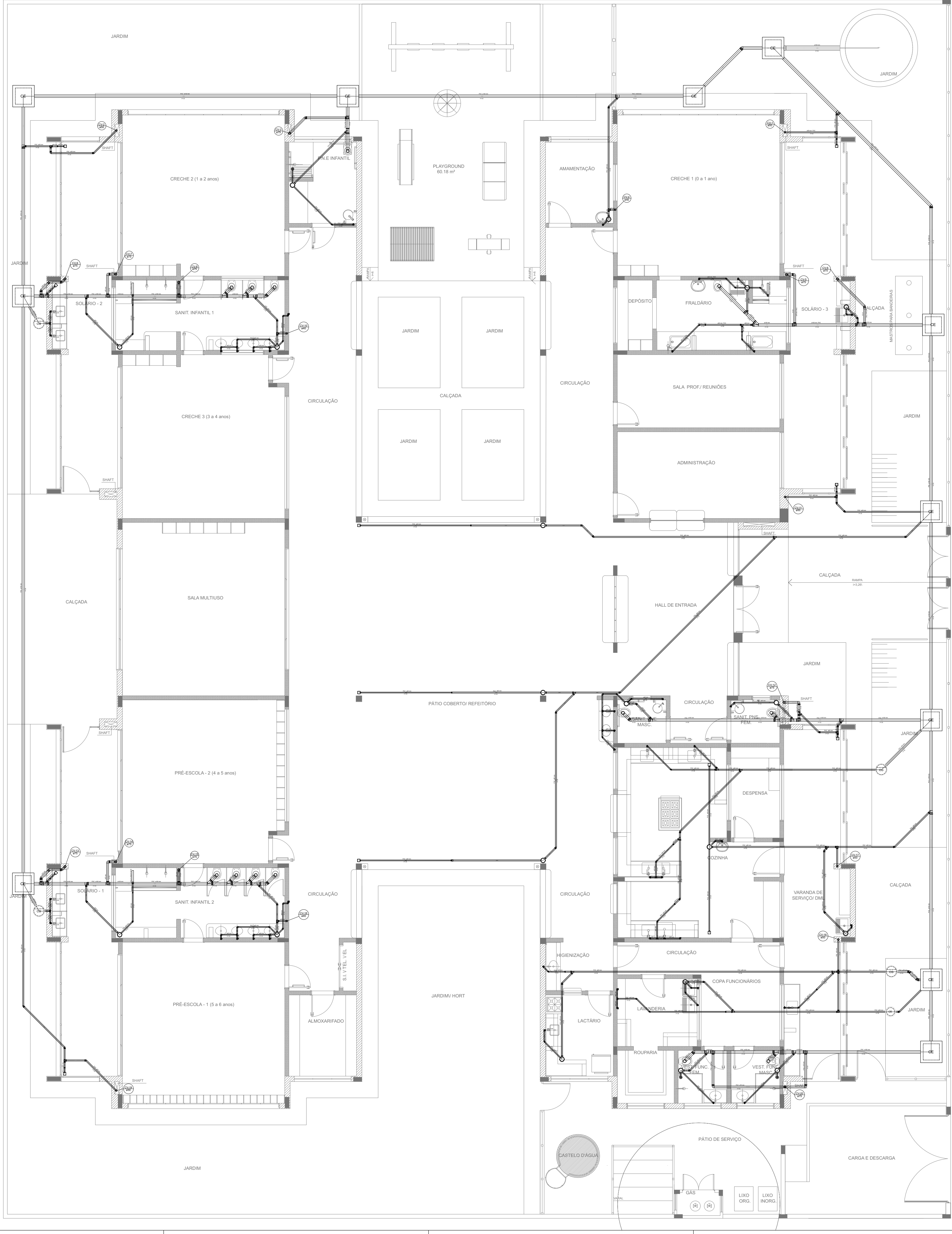
1 PLANTA BAIXA ESCALA 1/7
