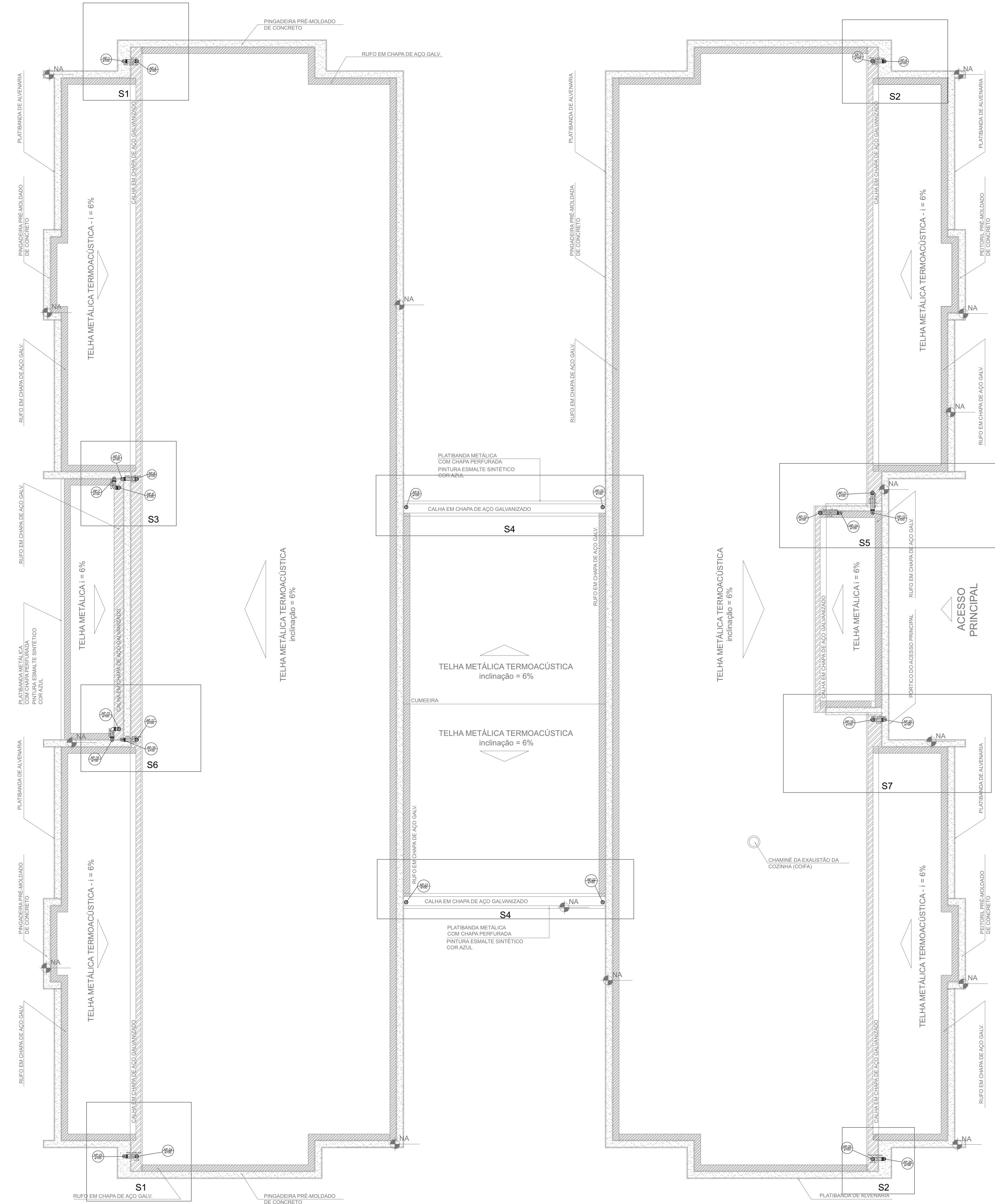
2 PLANTA DA COBERTURA - TRANSPOSIÇÃO ESCALA 1/7
