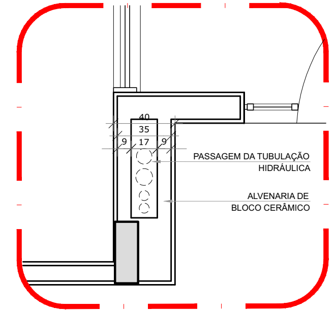
3 DETALHE - SHAFT HIDRÁULICA ESCALA 1/2
