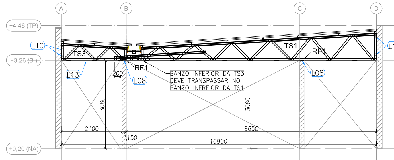
BLOCO B - ELEVÇÃO - EIXO 3, 4, 6, 7, 13, 14, 16 e 17 ESCALA: 1/75
