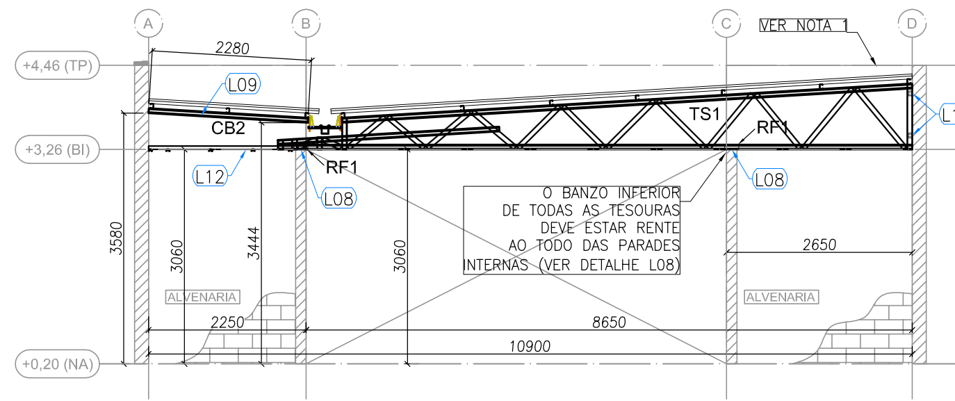
BLOCO B - ELEVÇÃO - EIXO 2, 8, 12 e 18 ESCALA: 1/75
