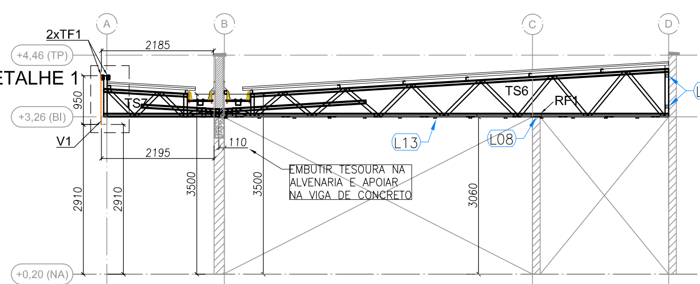
BLOCO B - ELEVÇÃO - EIXO 9, 10 e 11 ESCALA: 1/75
