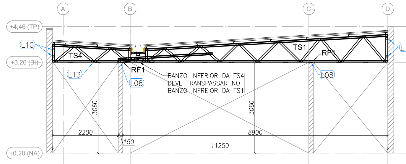
BLOCO B - ELEVÇÃO - EIXO 5 e 15 ESCALA: 1/75
