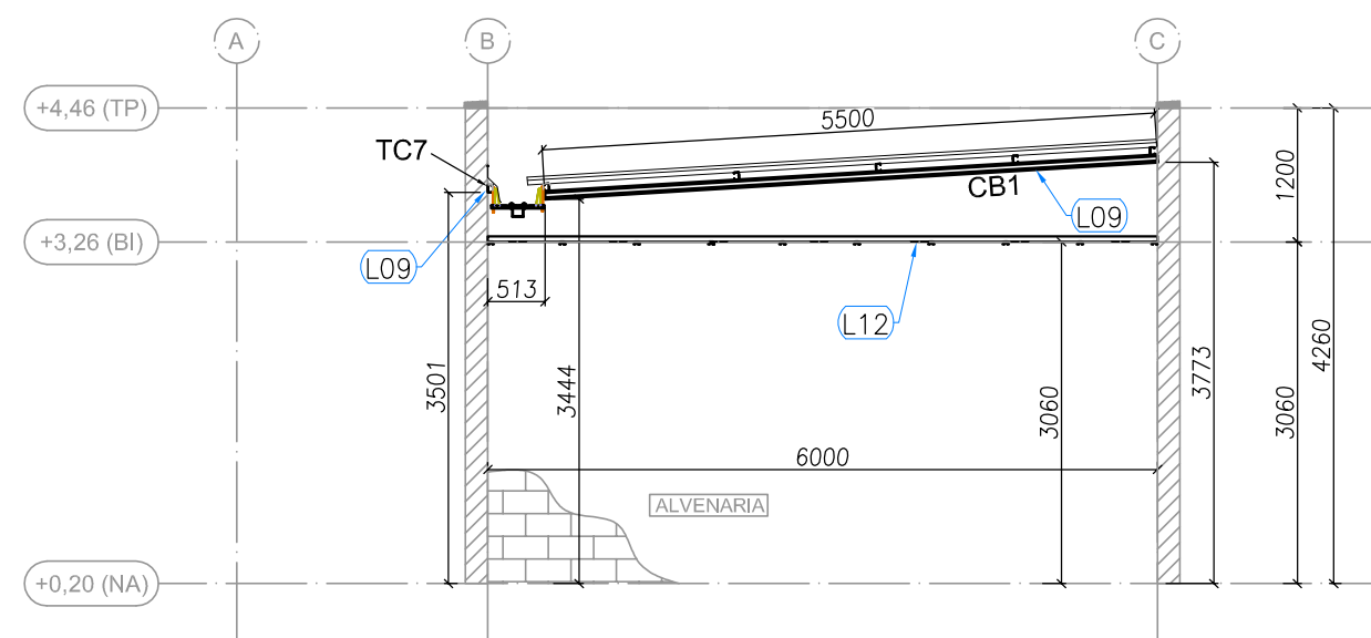
BLOCO B - ELEVÇÃO - EIXO 1 e 19 ESCALA: 1/75
