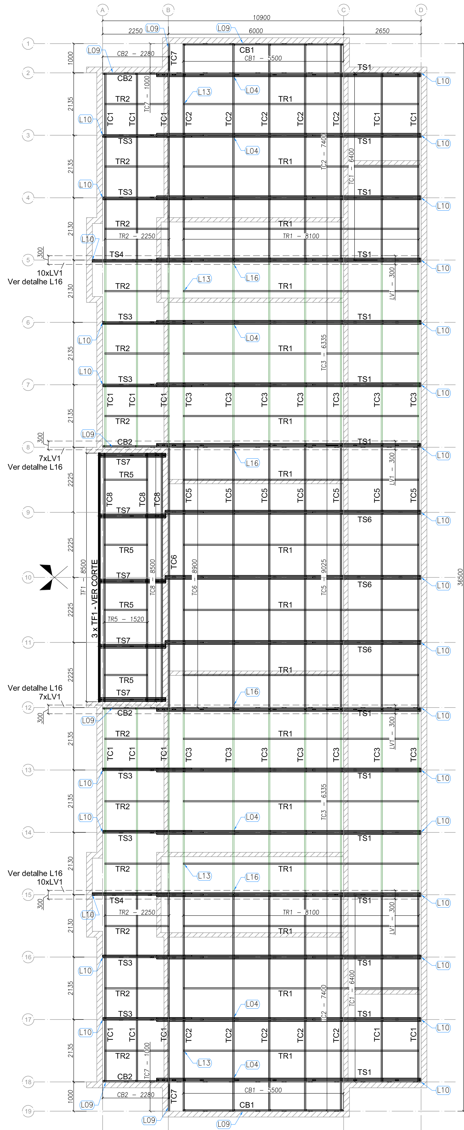
BLOCO B - PLANTA DE COBERTURA - CAIBROS, TESOURAS, TERÇAS, TRAVAMENTOS e LUVAS ESCALA: 1/75
