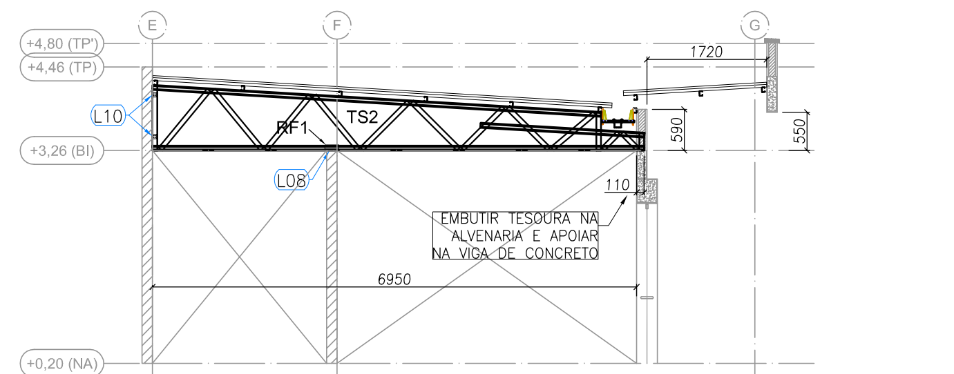
7 BLOCO A - ELEVACÃO - EIXO 9, 10 e 11 ESCALA: 1/75
