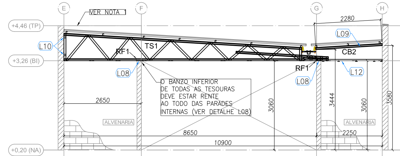
4 BLOCO A - ELEVACÃO - EIXO 2, 8, 12 e 18 ESCALA: 1/75
