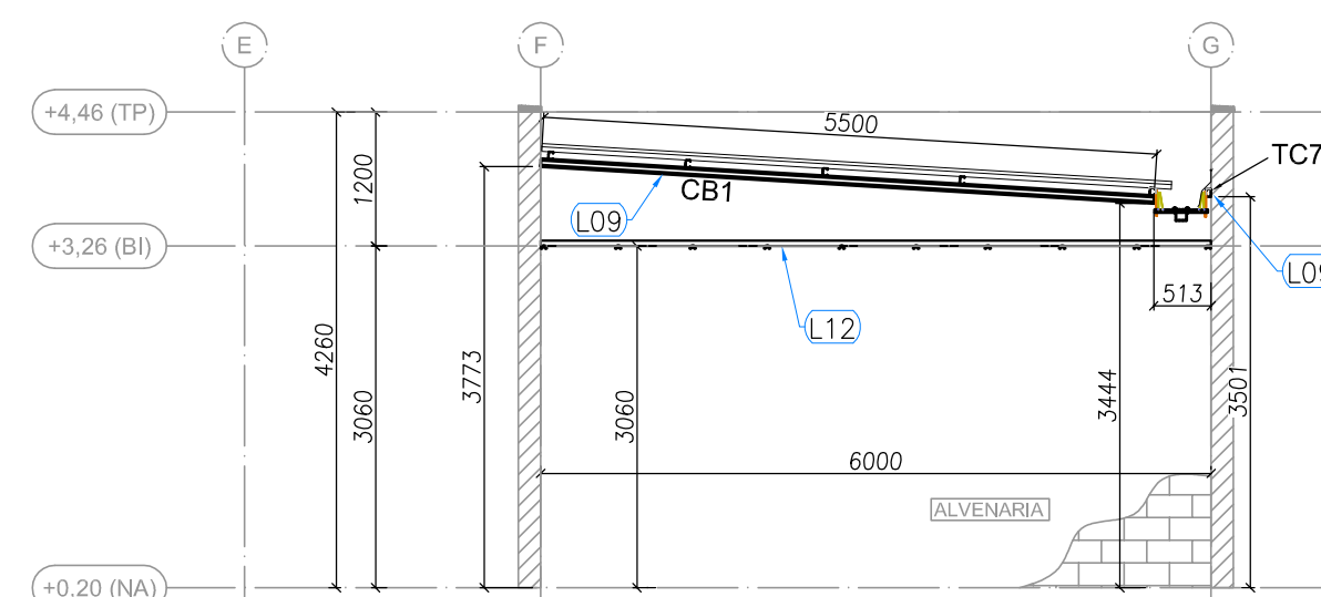
3 BLOCO A - ELEVACÃO - EIXO 1 e 19 ESCALA: 1/75
