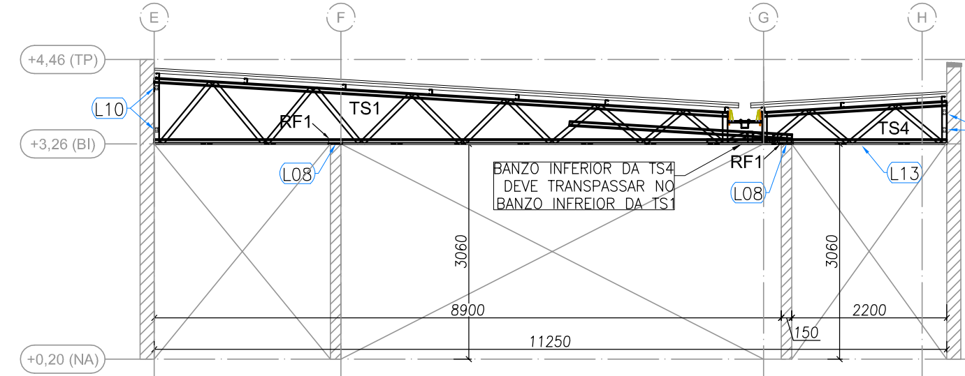
6 BLOCO A - ELEVACÃO - EIXO 5 e 15 ESCALA: 1/75
