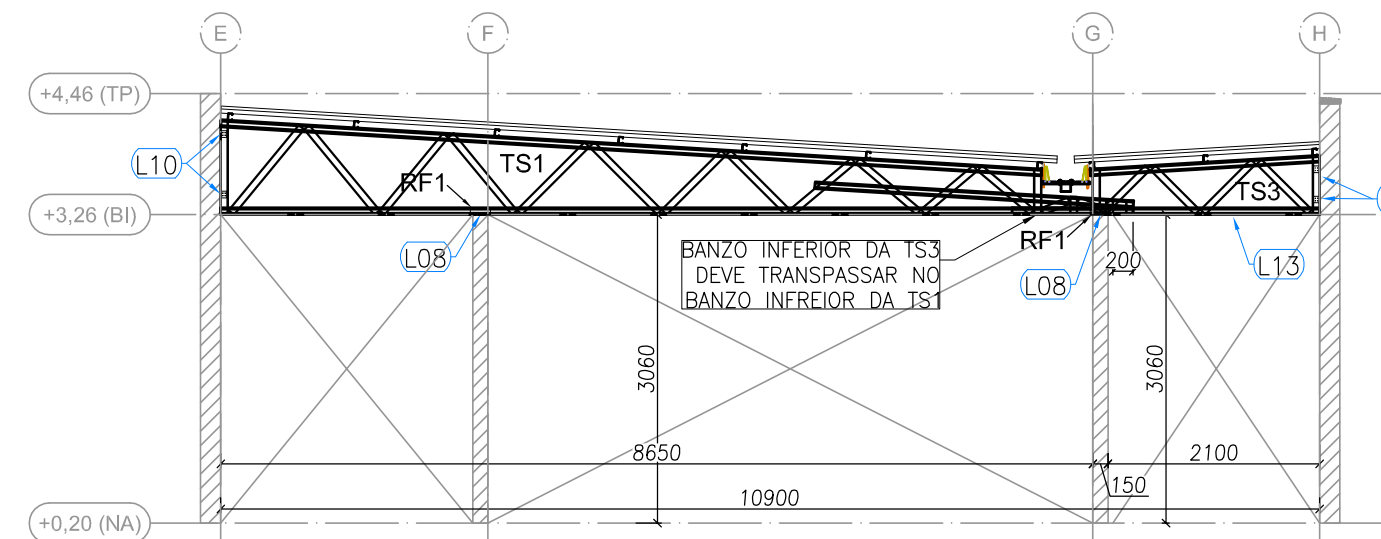
5 BLOCO A - ELEVACÃO - EIXO 3, 4, 6, 7, 13, 14, 16 e 17 ESCALA: 1/75
