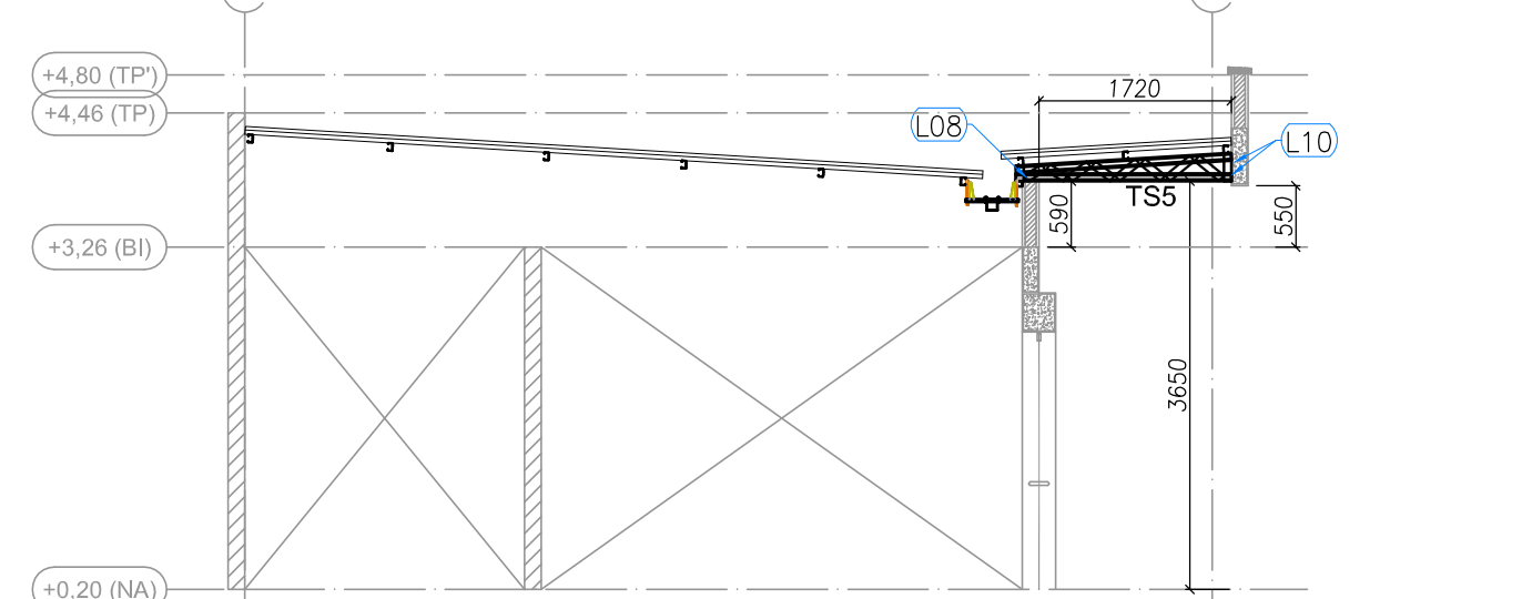
7 BLOCO A - ELEVACÃO - EIXO 10' e 10'' ESCALA: 1/75
