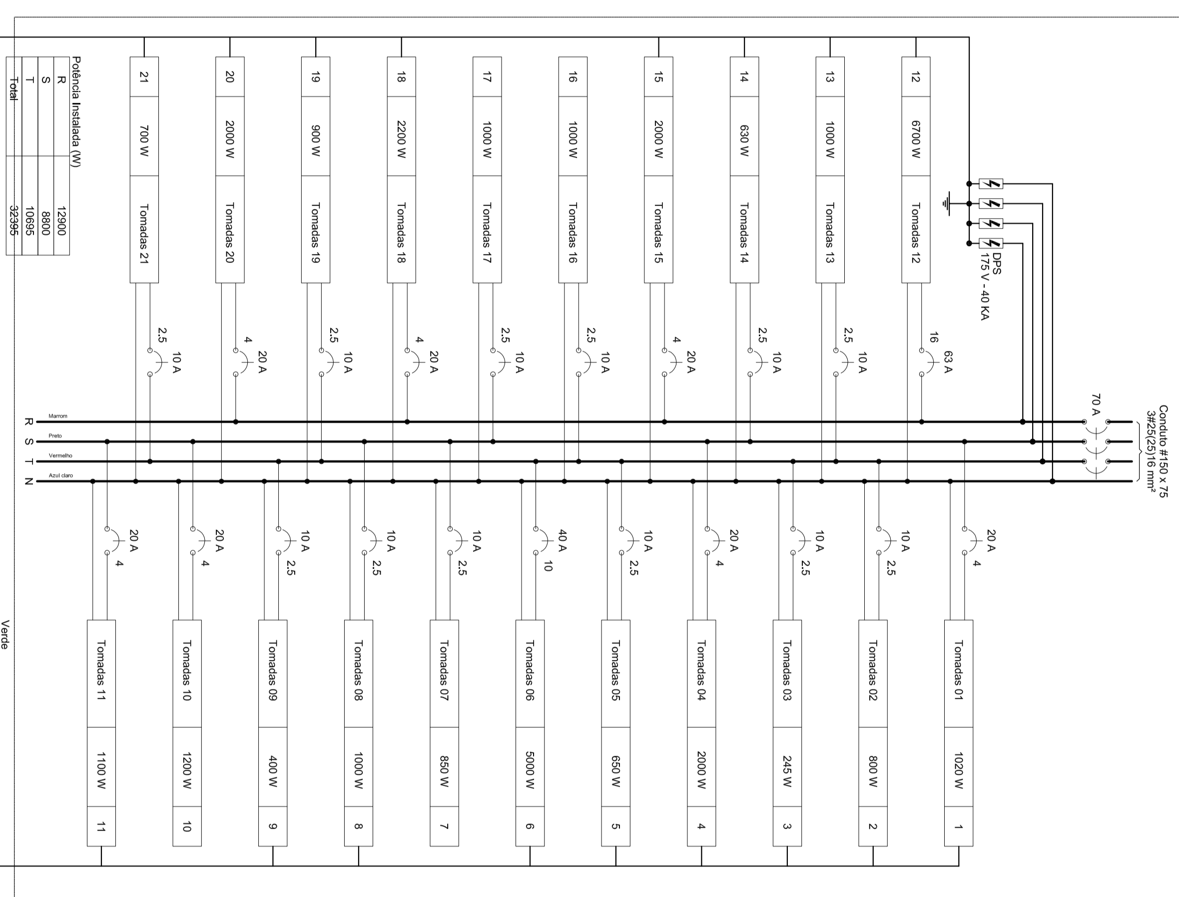
Q05 (Quadro de Distribuição Tomada - 05)
