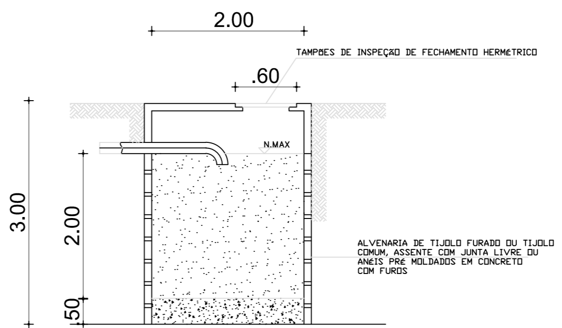
DETALHE POÇO ABSORVENTE
