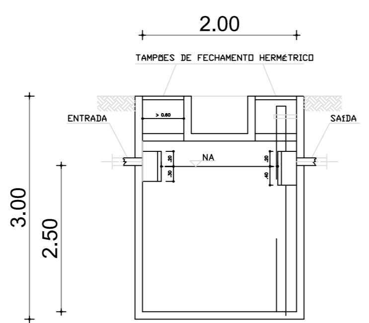
DETALHE FOSSA SEPTICA
