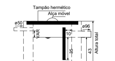
Caixa de gordura - TÉRREO Corte 1 - ESC. 1:25
