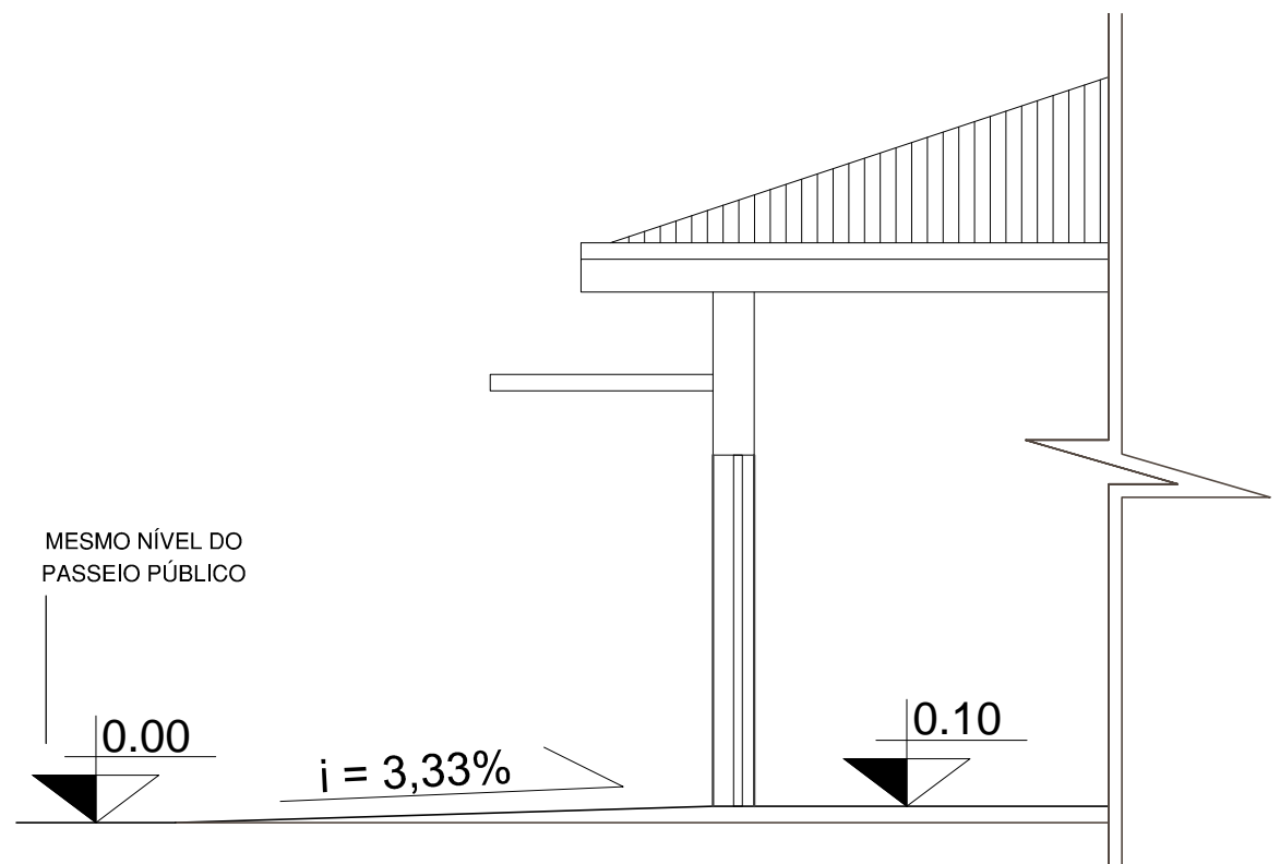
PERFIL RAMPA DE ACESSIBILIDADE Esc. 1/50
