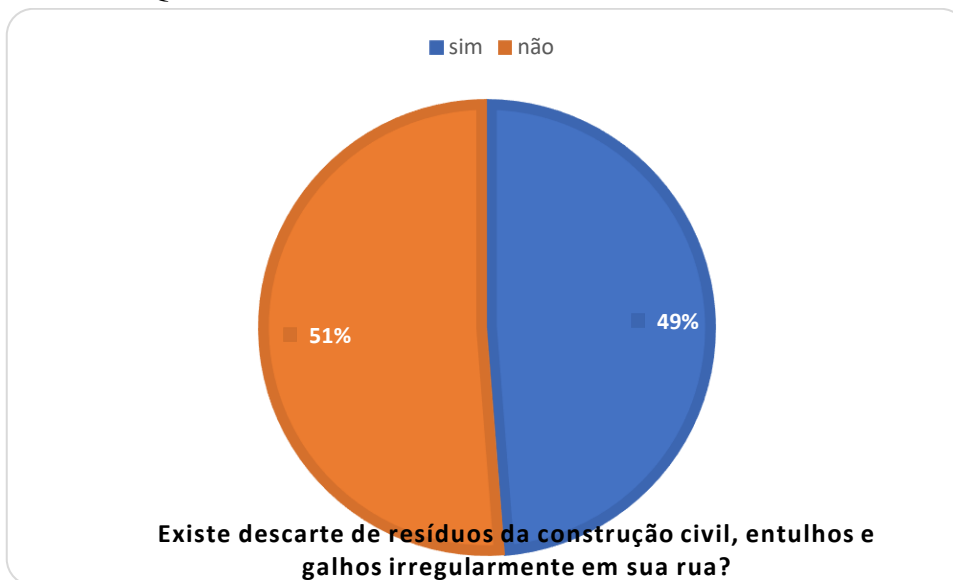
Gráfico 8: Questionário SRSU
