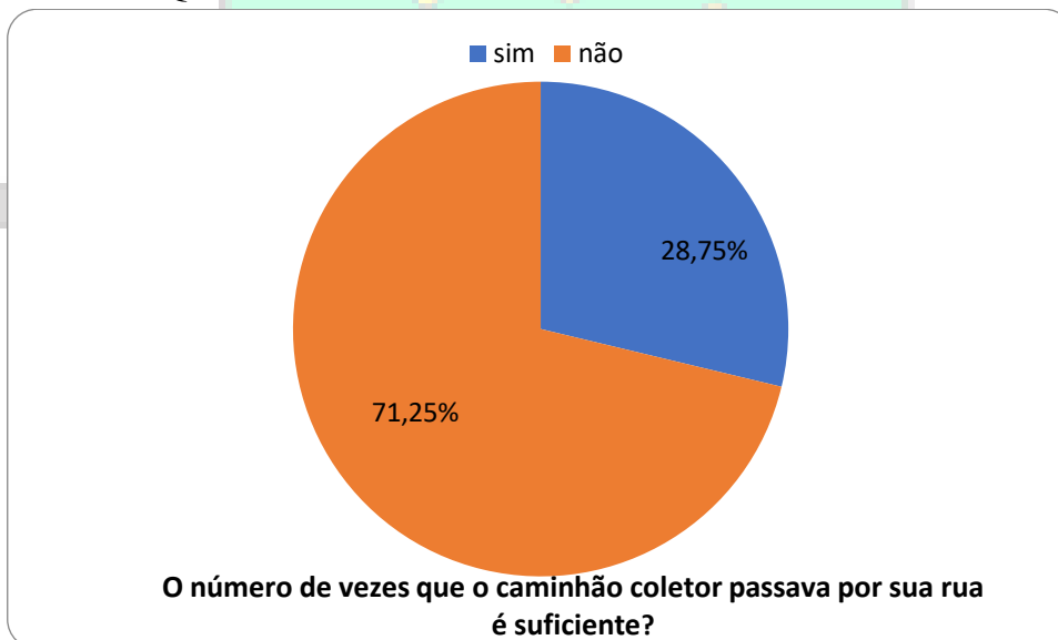
Gráfico 7: Questionário SRSU
