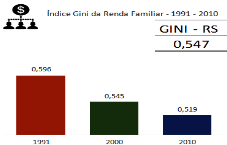
Figura 15: Índice GINI
