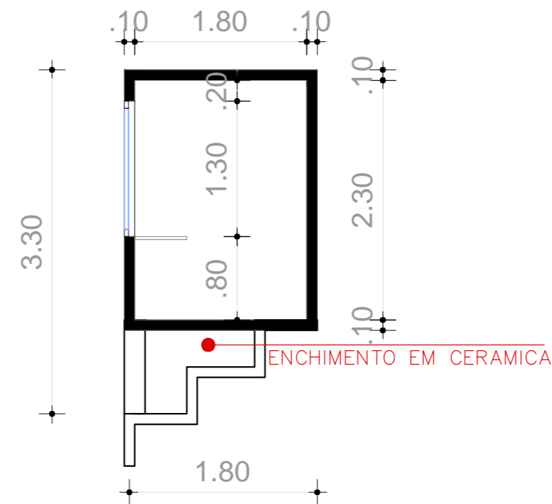
04 Corte ESC: 1/50
