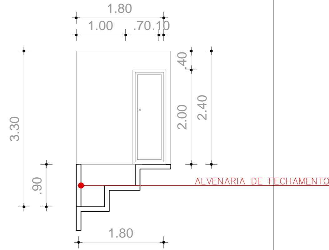
02 Fachada Lateral ESC: 1/50
