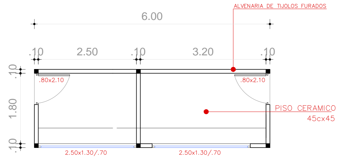
01 Planta Baixa ESC: 1/50 Área: 12.00 m 2
