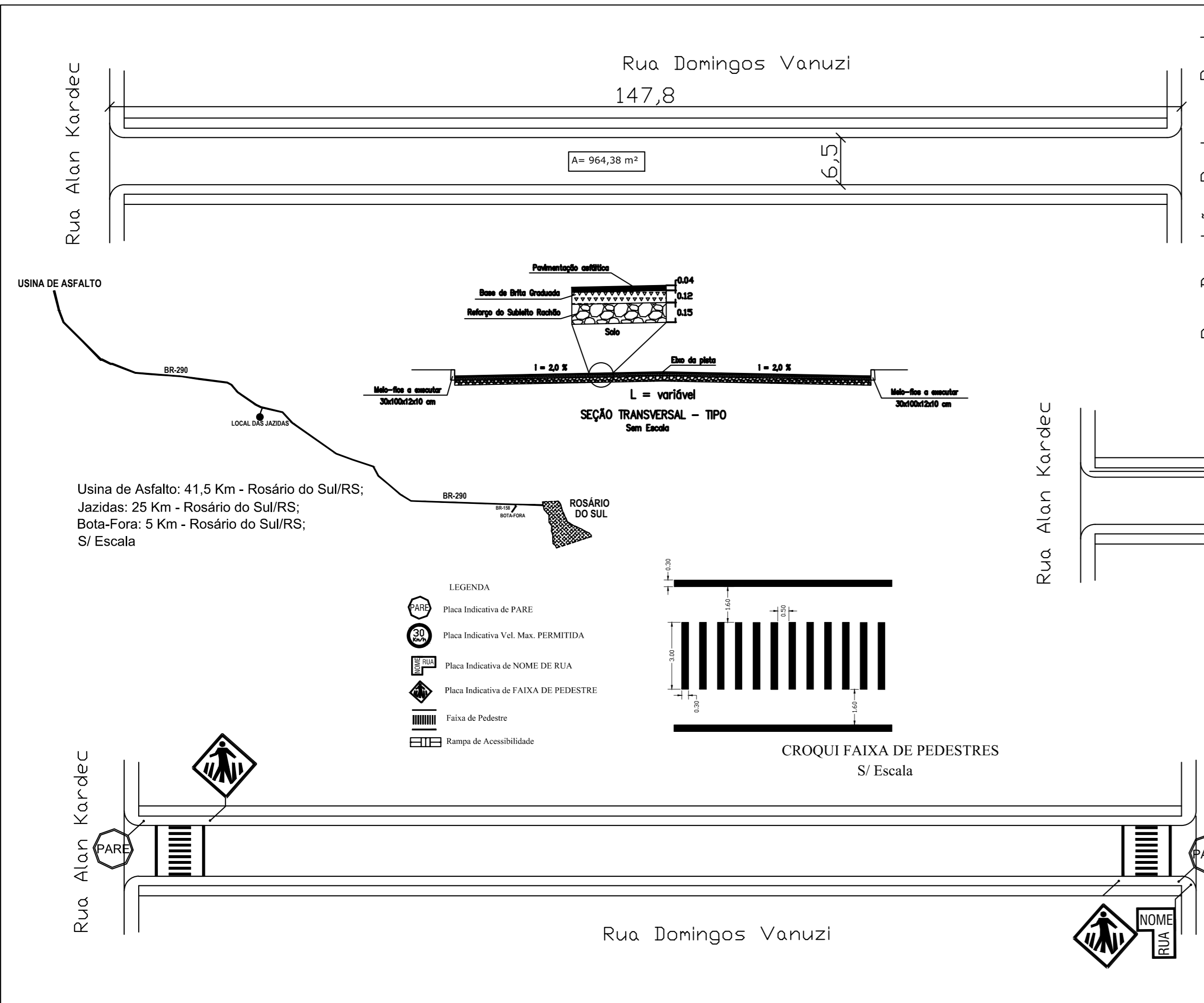
Planta Baixa Pavimentação Asfáltica Esc. 1:50
